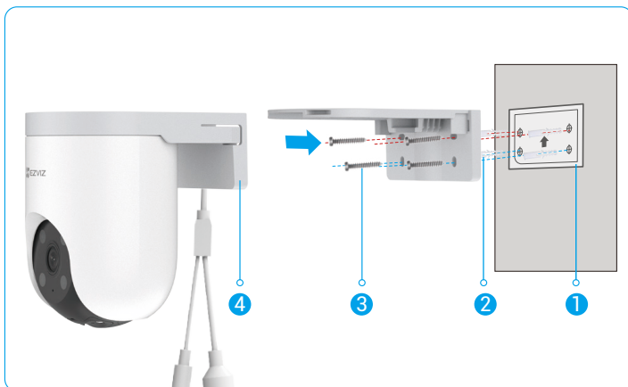
Fig. 2 Montage mural
